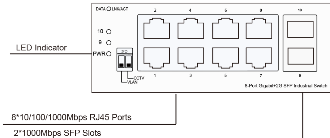
图 2-1 交换机前面板示意图
