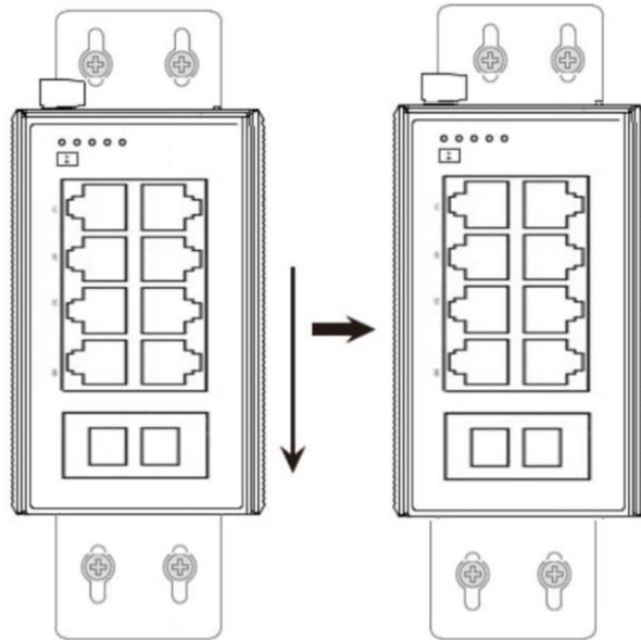
工业机壁挂式安装示意图
